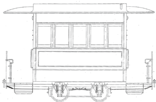
▲株式会社千住馬車鉄道会社車台図
